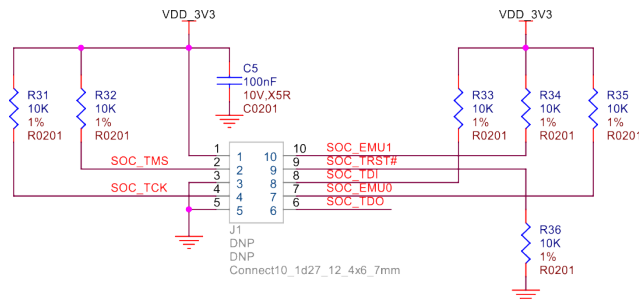
Fig. 3.43: TagConnect (JTAG)
