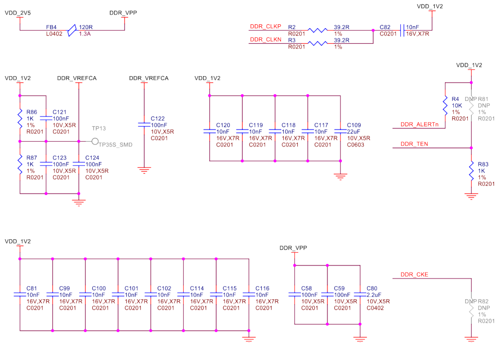
Fig. 3.39: DDR power
